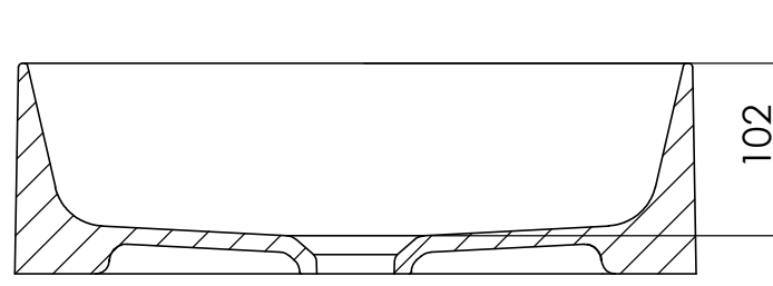
SEZIONE B-B
